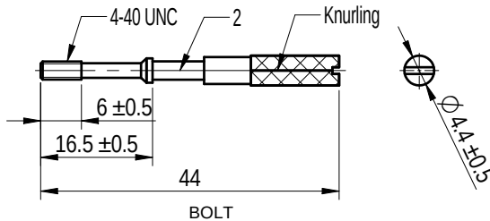
BOLT
