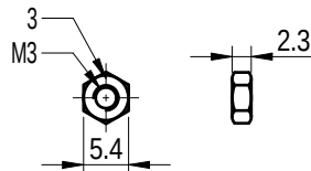
NUT
