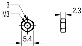
NUT
