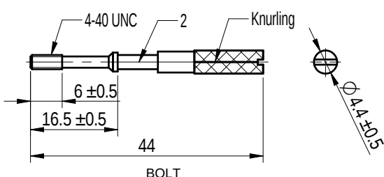
BOLT
