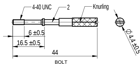
BOLT
